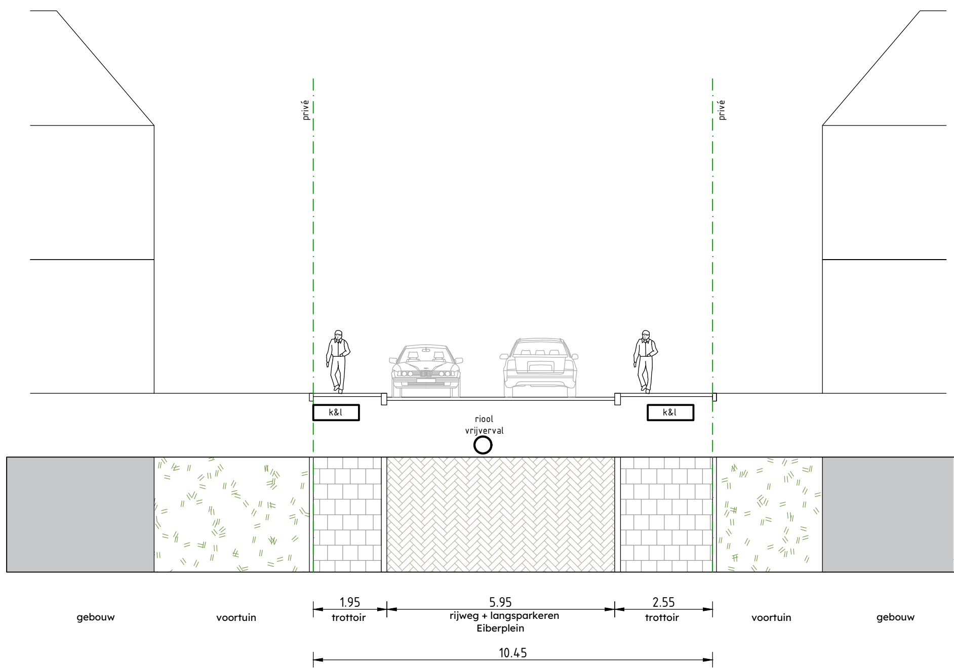
DOORSNEDE 1 | HUIDIGE SITUATIE
