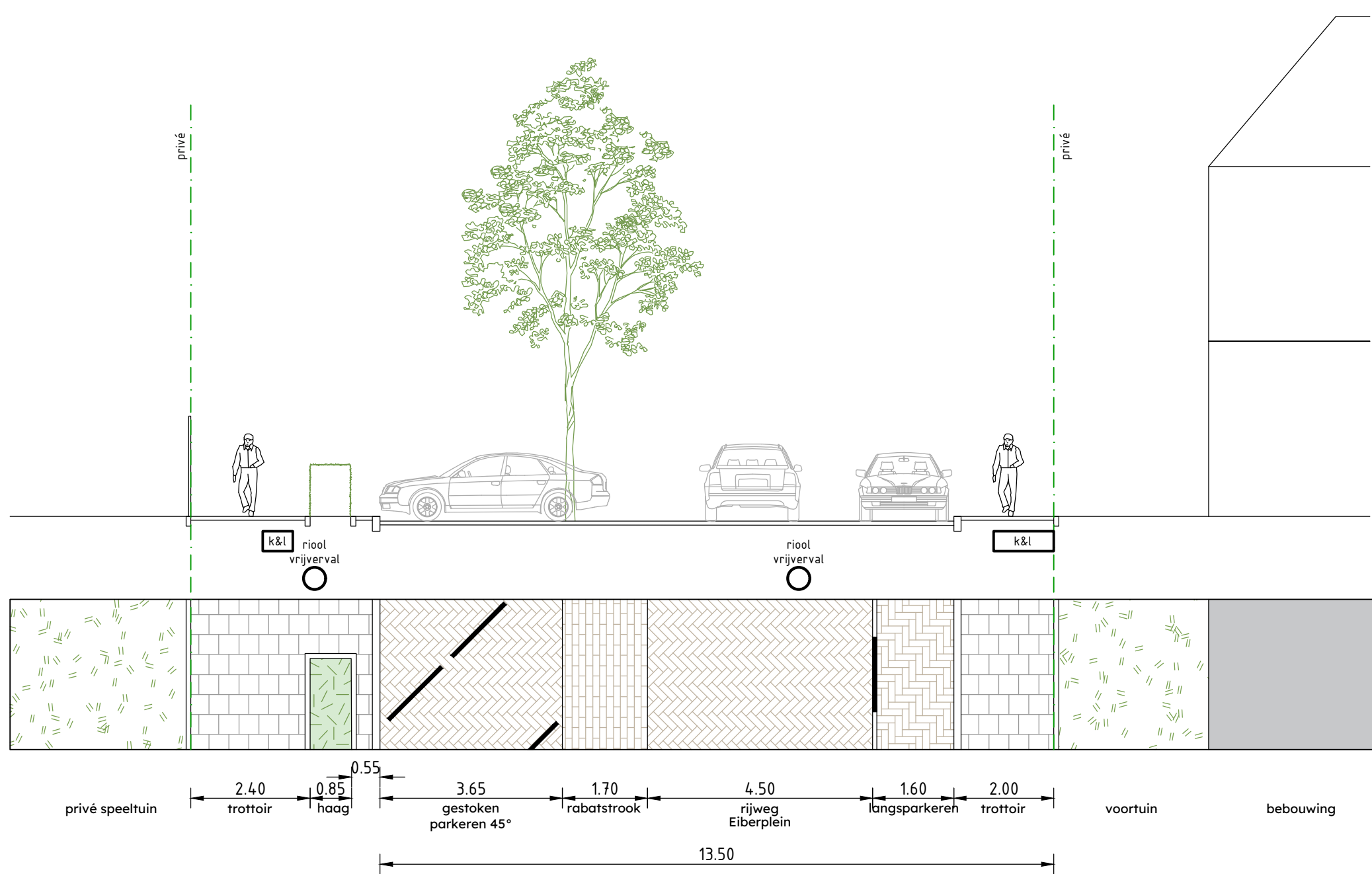
DOORSNEDE 2 | HUIDIGE SITUATIE
