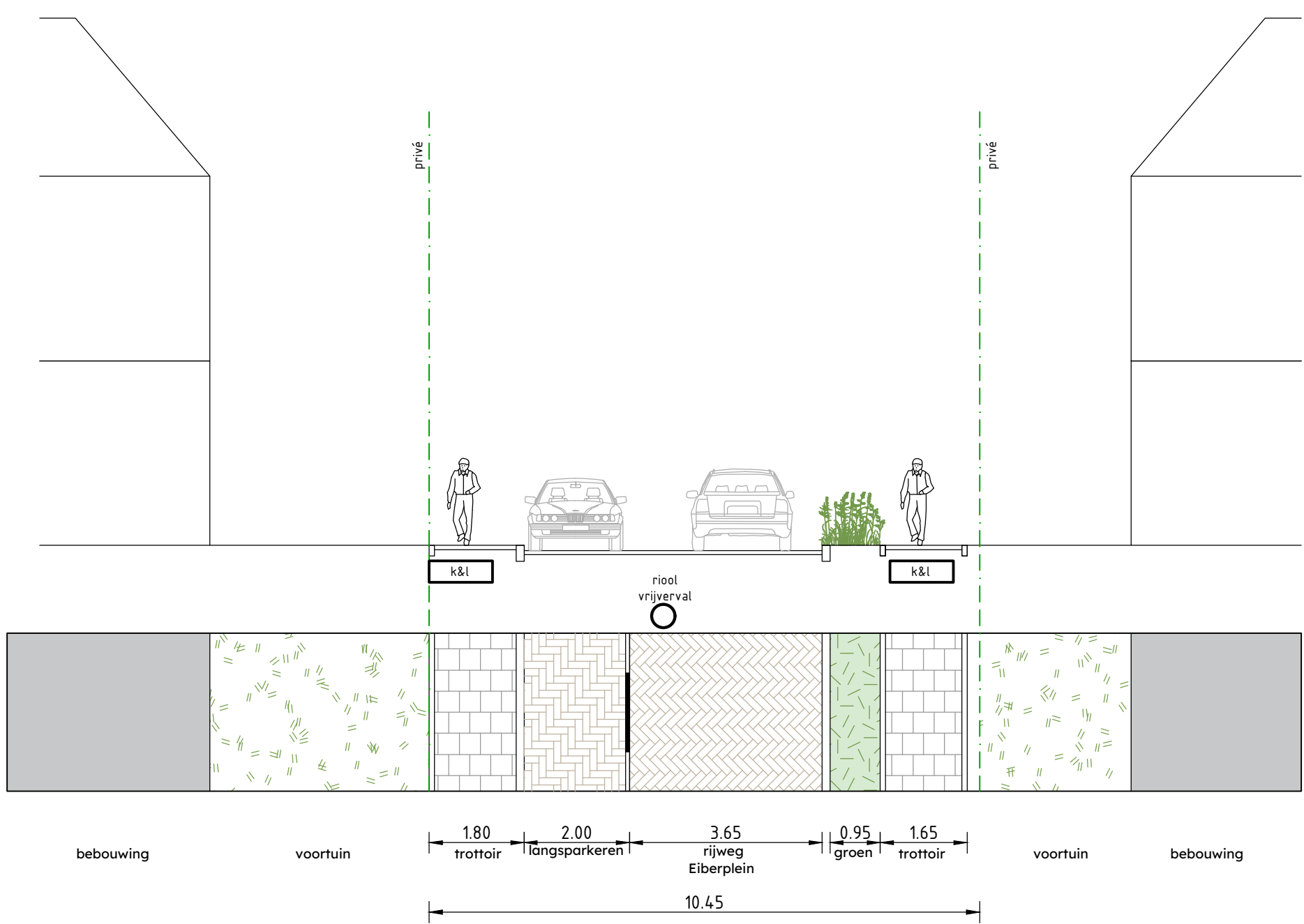
DOORSNEDE 1 | NIEUWE SITUATIE
