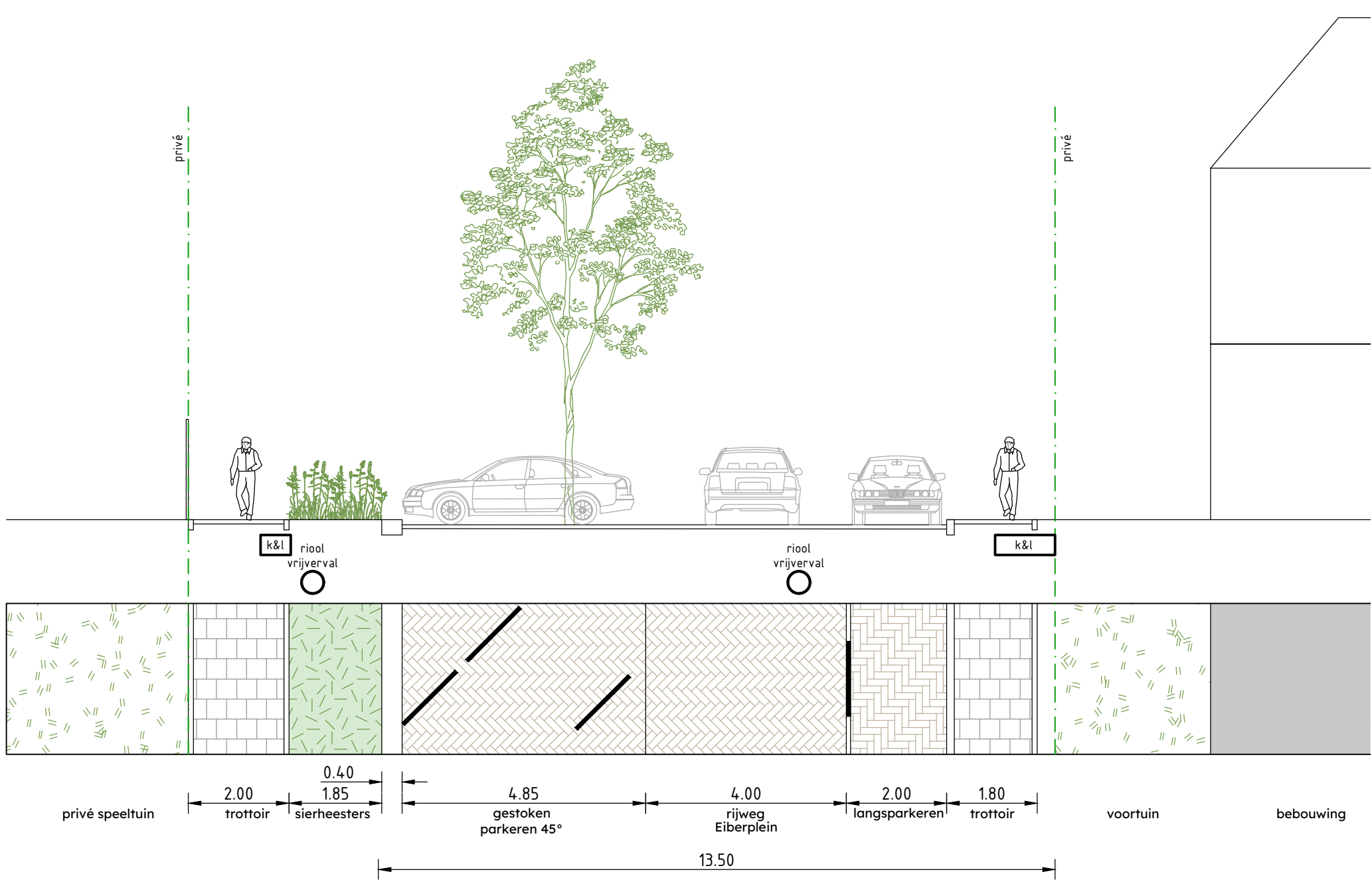
DOORSNEDE 2 | NIEUWE SITUATIE
